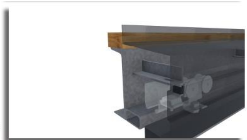
Detail regenkap bovenrollende deur bij montage op vlakke gevel
